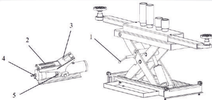
ФИКСИРУЮЩИЙ РЫЧАГ (1)
