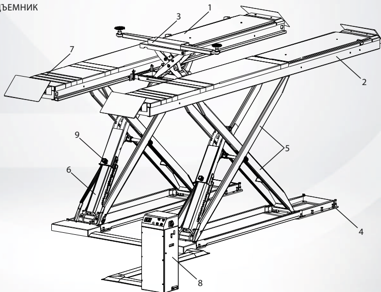
Рис.2 ПОДЪЕМНИК
